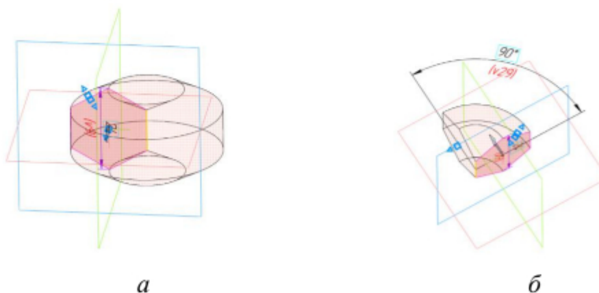
Рис. 6 Варианты выполнения операции «Вращение»: a – на угол 360^{\circ} , б – на заданный угол
