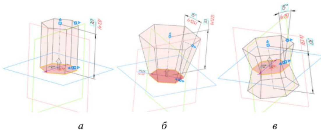
Рис. 5 Варианты выполнения операции «Выдавливание»: a – перпендикулярно плоскости эскиза, б – на заданный угол, в – симметрично плоскости эскиза
