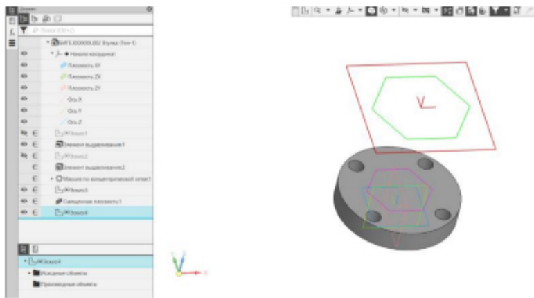
Рис. 20 Эскиз на смещенной плоскости
