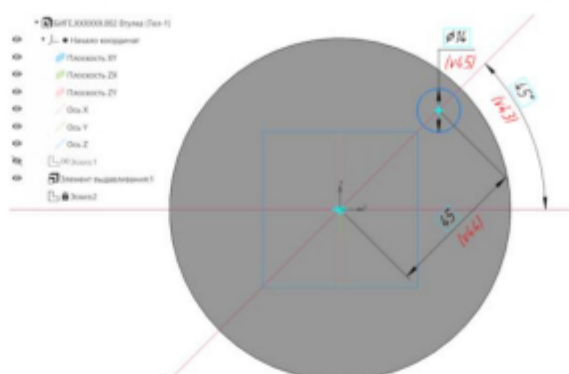
Рис. 15 Эскиз для команды «Вырезать выдавливанием»
